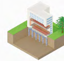
Pompe à chaleur sur géostructures énergétiques
